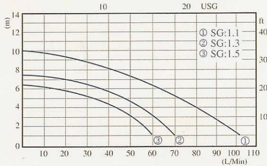
NH-200PS 50Hz Nominal speed 2,700 r.p.m
