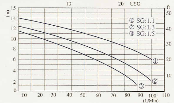
NH-250PS 60Hz Nominal speed 3,350 r.p.m
