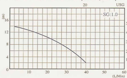
NH-200PS-F-Z 50Hz Nominal speed 2,500 r.p.m
