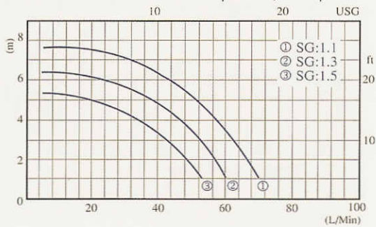
NH-200PS-F 50Hz Nominal speed 2,500 r.p.m
