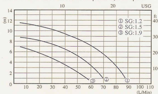
NH-250PS-F 50Hz Nominal speed 2,700 r.p.m
