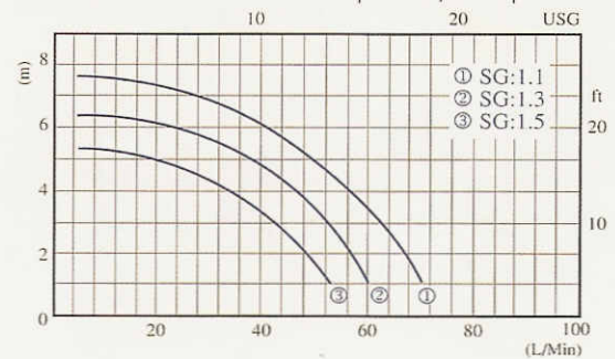
NH-200PS-F 60Hz Nominal speed 3,300 r.p.m
