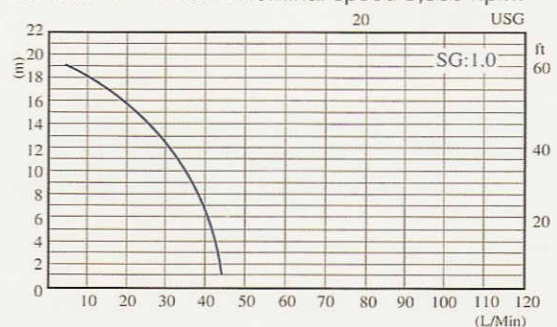
NH-200PS-F-Z 60Hz Nominal speed 3,300 r.p.m
