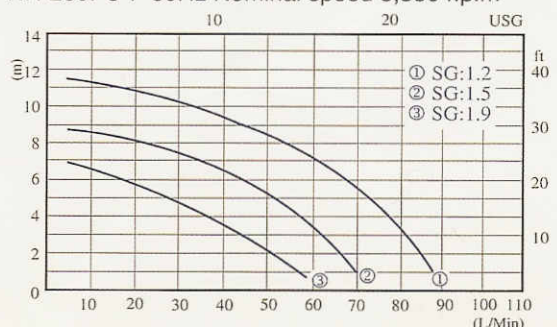
NH-250PS-F 60Hz Nominal speed 3,350 r.p.m
